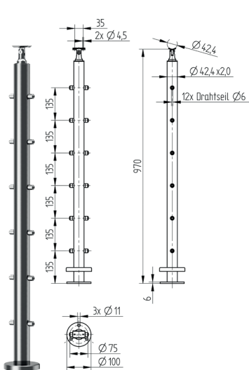
Geländerpfosten Drahtseil, Mitte, aufgesetzt für Drahtseil Ø 6 mm
