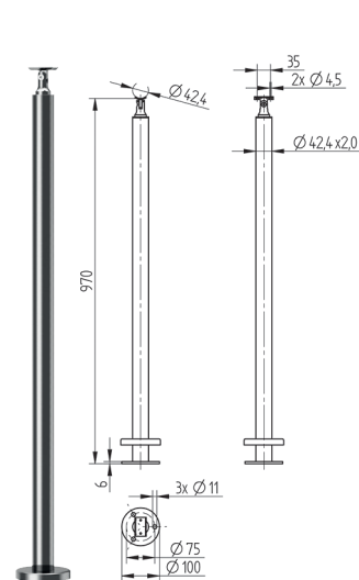
Geländerpfosten, aufgesetzt
