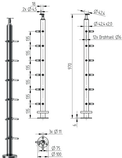
Geländerpfosten Drahtseil, Ecke, aufgesetzt für Drahtseil Ø 6 mm
